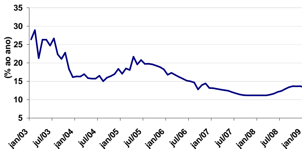
Gráfico VI.1 - Taxa Selic
